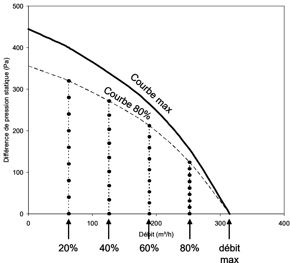
Figure 2: Points de mesure pour le réglage automatique des ventilateurs
