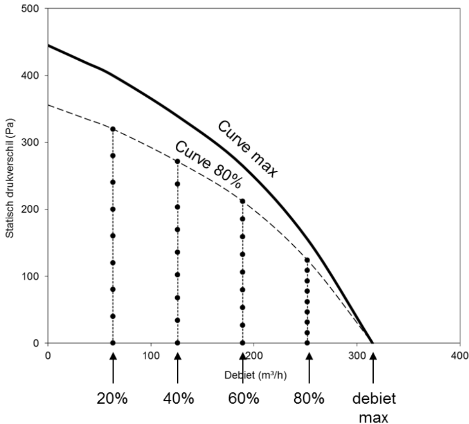
Figuur 2: Meetpunten voor automatische regeling van ventilatoren
